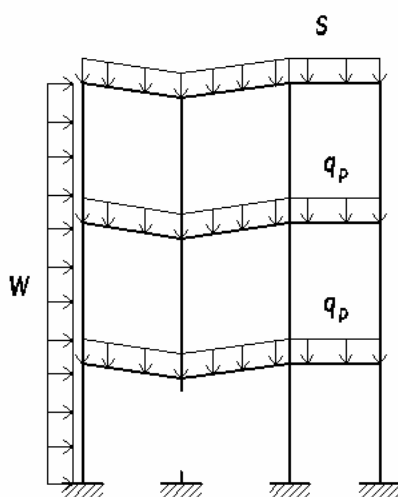
Рис. 7 Расчетная схема МГСН
