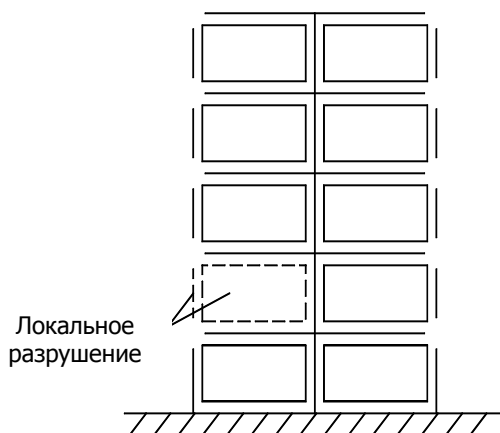
Рис. 6 Расчетная схема локального обрушения
