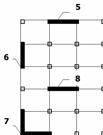
Рис. 19 Схема стен
